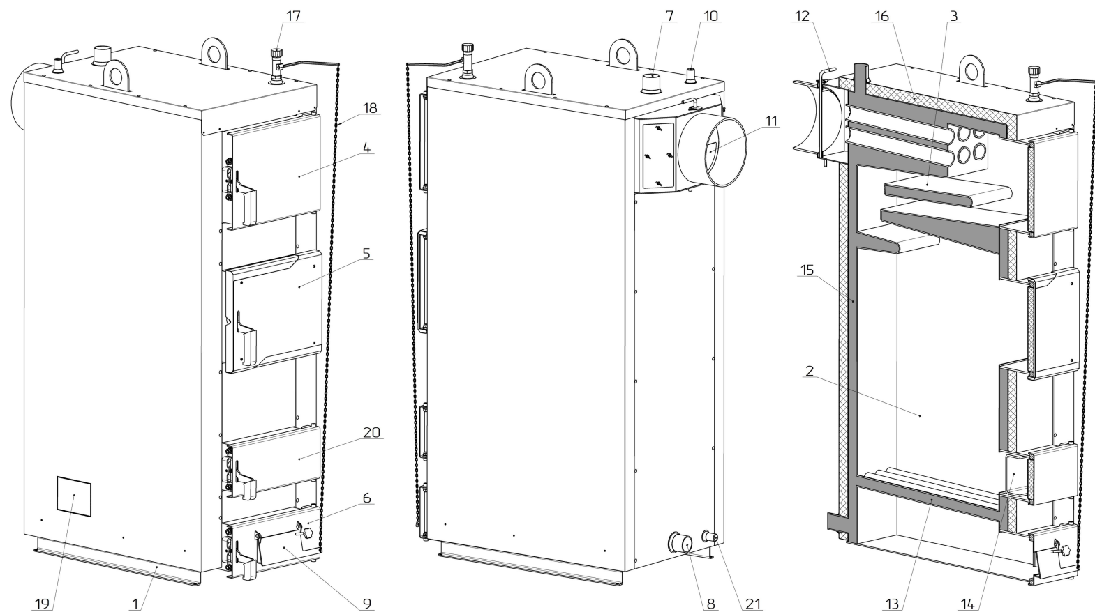
Figura 2b – Elementele principale ale cazanului Altep-Compact (50-95 kW)
