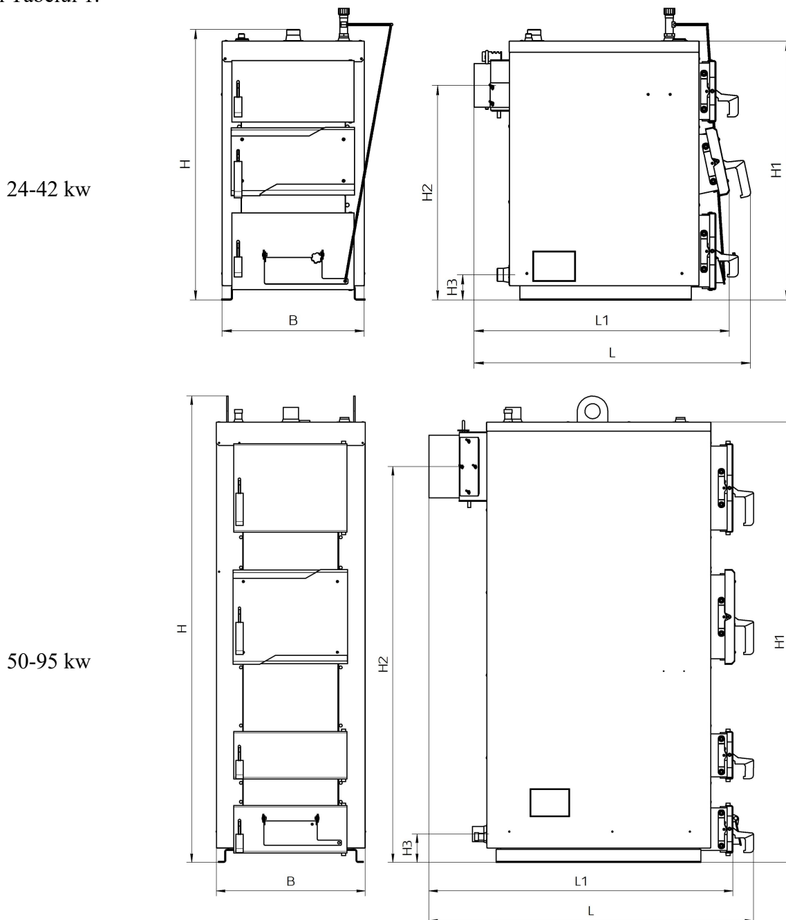
Figura 1 – Desen dimensional al cazanului Altep-Compact
