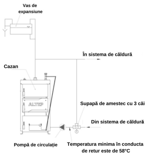
Figura 4 – Scheme de conectare a cazanului la sistemul de încălzire
