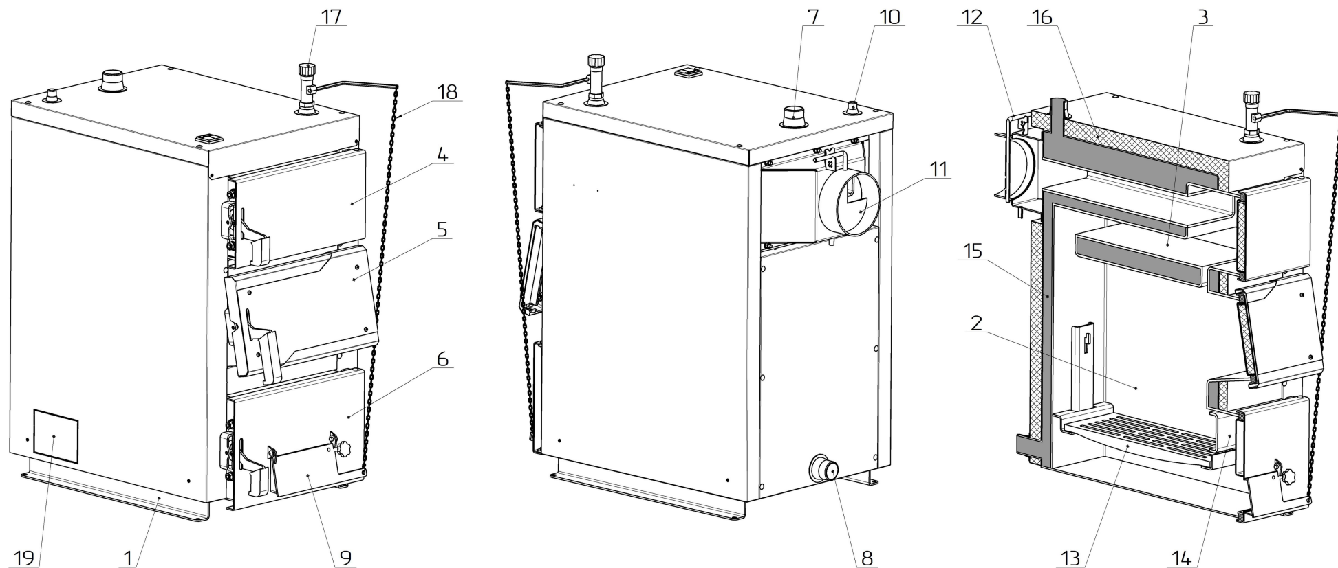
Figura 2a – Elementele principale ale cazanului Altep-Compact (24-42 kW)
